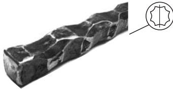
R 118/A/1 12x3000 mm 1770 Ft R 118/A/2 14x3000 mm 2740 Ft Él és lapkovácsolt négyzetacél
